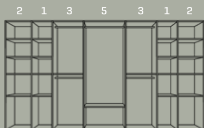
360-390 CM 4 SKAPDØRER NR. 360390
