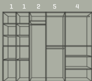
250-280 CM 2 ELLER 3 SKAPDØRER NR. 250280
