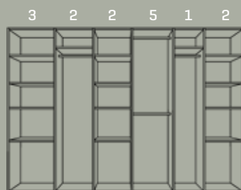
285-315 CM 3 SKAPDØRER NR. 285315
